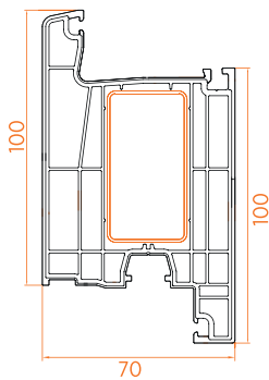
Geniş Kapı Profili
