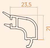
■ 24 mm Çift Cam Çıtası
