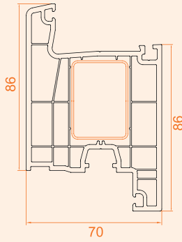
Kapı Kanat Profili / 4 Odacık
