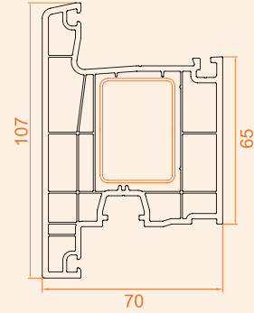
Dışa Açılım Kapı / 4 Odacık
