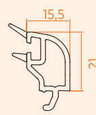
■ 32 mm Üç Cam Çıtası
