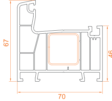
Kasa Profili / 5 Odacık
