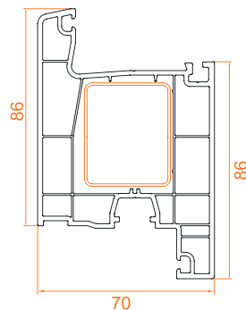
Kapı Kanat Profili / 3 Odacık
