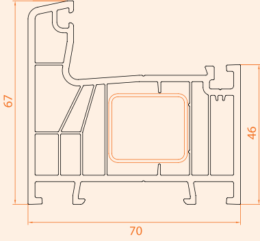
Kasa Profili / 6 Odacık
