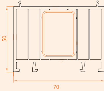
■ Kasa Yükseltme Profili / 50 mm
