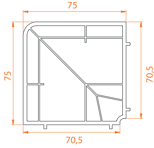
■ 90 Derece Köşe Profili
