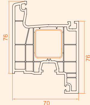
Dar Kapı Profili
