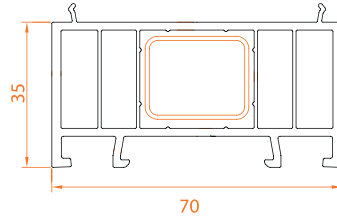
■ Kasa Yükseltme Profili / 35 mm
