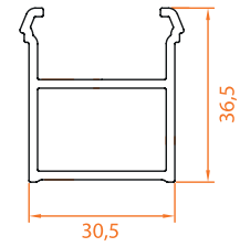
■ Kasa Montaj Profili
