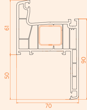
Pervazlı Kasa Profili / 5 Odacık
