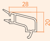
■ 20 mm Çift Cam Çıtası
