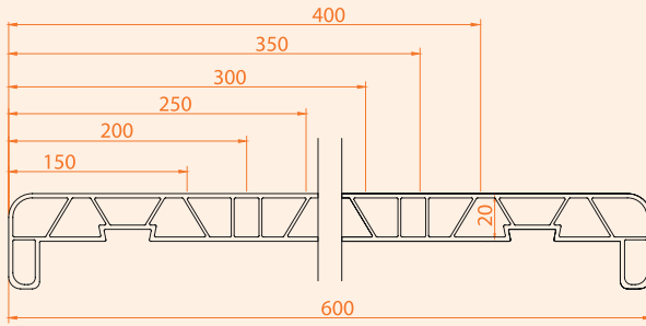
■ UPVC Denizlik Profili / 600 mm
