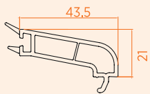
■ 4 mm Tek Cam Çıtası
