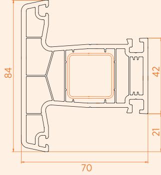
Orta Kayıt Profili / 5 Odacık
