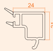
■ 24 mm Kare Çıta
