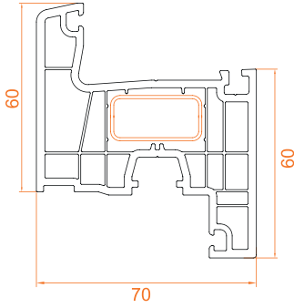
Kanat Profili / 5 Odacık
