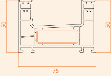
Kasa Profili / Çift Raylı
