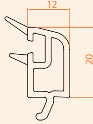
■ 20 mm Çift Cam Çıtası
