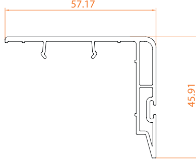
■ Kanat Kapama Profili
