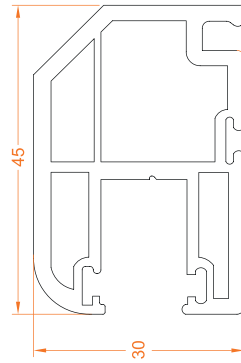
Sineklikli Kanat Profili
