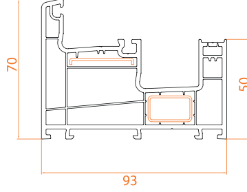
Kasa Profili / Tek Raylı
