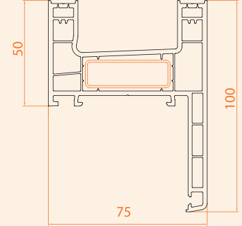
Pervazlı Kasa Profili / Çift Raylı
