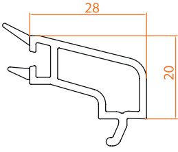
■ 4 mm Tek Cam Çıtası
