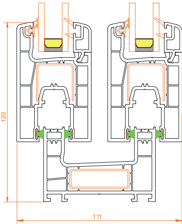
■ Çift Ray Montajı
