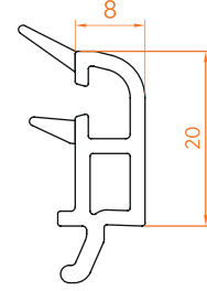
■ 24 mm Çift Cam Çıtası
