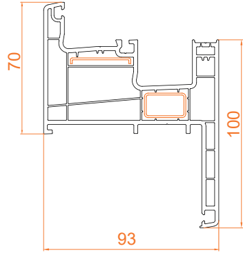
Pervazlı Fix Kasa Profili / 4 Odacık
