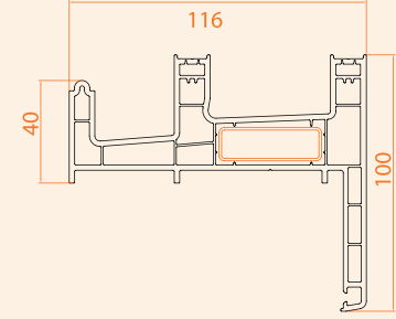
Kasa Profili; Çift Raylı, Sineklikli, 40 mm Pervazlı
