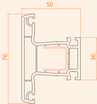
Orta Kayıt Profili
