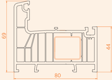
Kasa Profili / 8 Odacık
