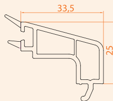
20 mm Düz Cam Çıtası
