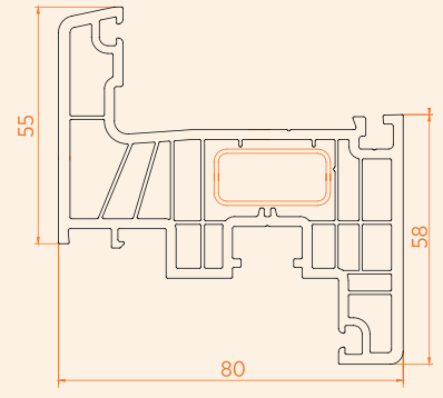
Kanat Profili / 7 Odacık
