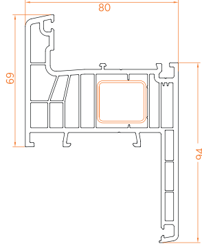
Pervazlı Kasa Profili / 8 Odacık
