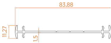
■ İnce Bağ Profili
