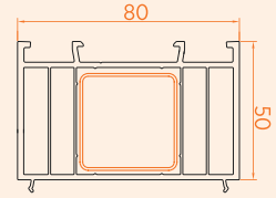
■ Kasa Yükseltme Profili / 50 mm
