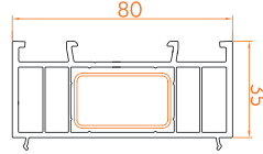
■ Kasa Yükseltme Profili / 35 mm
