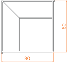
■ 90 Derece Köşe Profili
