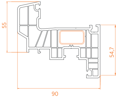
Damlalıklı Kanat / 8 Odacık
