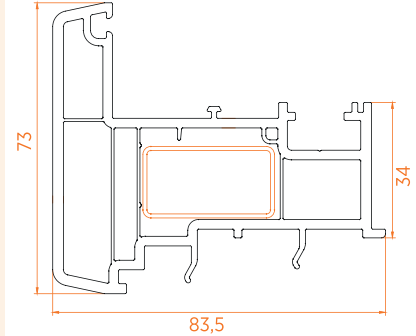
Hareketli Orta Kayıt Profili
