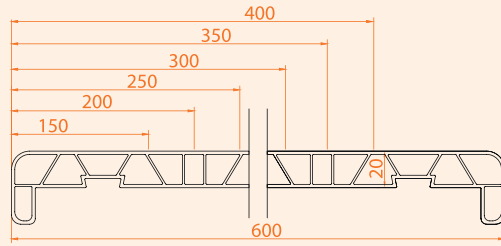
■ UPVC Denizlik Profili / 600 mm
