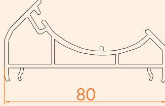
■ Açılı Dönüş Adaptörü / 80 mm
