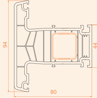
Orta Kayıt Profili / 7 Odacık
