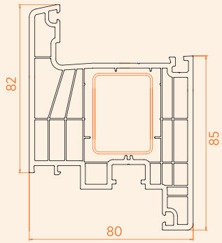
Kapı Kanat Profili / 6 Odacık
