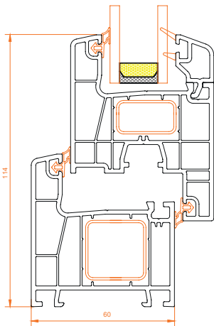
Pencere Montajı
