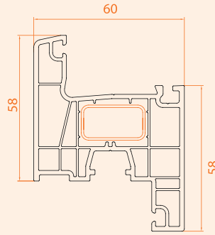
Kanat Profili / 4 Odacık
