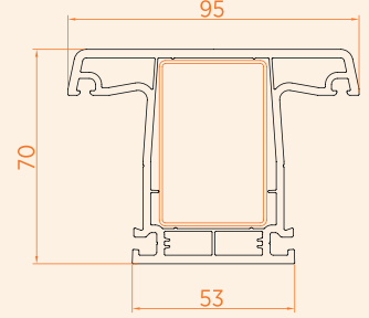
■ Yalıtımlı Sürme Orta Kayıt Profili
