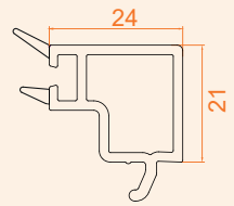
■ 24 mm Kare Çıta
