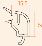
■ 32 mm Üç Cam Çıtası
