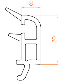
■ 24 mm Çift Cam Çıtası
