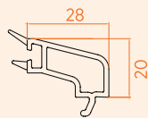
■ 20 mm Çift Cam Çıtası
