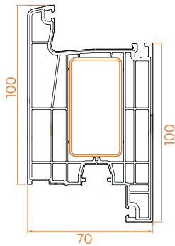
Geniş Kapı Profili
