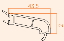
■ 4 mm Tek Cam Çıtası
