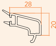
■ 20 mm Çift Cam Çıtası
